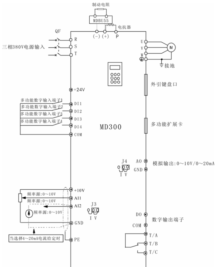
图 3-8 75kW/90kW 变频器接线图
