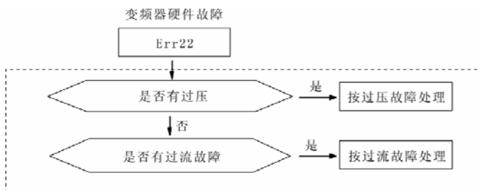
图 8-18 变频器硬件故障 (Err22)
