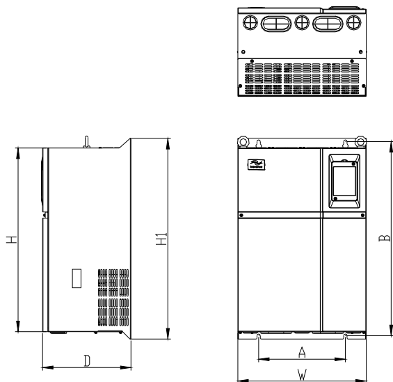
图 2-9 MD300N 系列 18.5kW~90kW 外形尺寸及安装尺寸示意图
