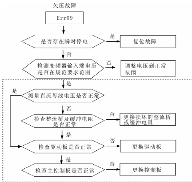
图 8-9 欠电压故障 (Err09)
