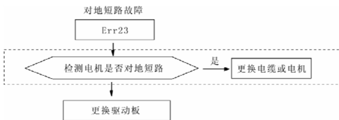
图 8-19 对地短路故障 (Err23)
