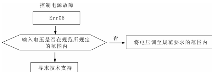
图 8-8 控制电源故障 (Err08)
