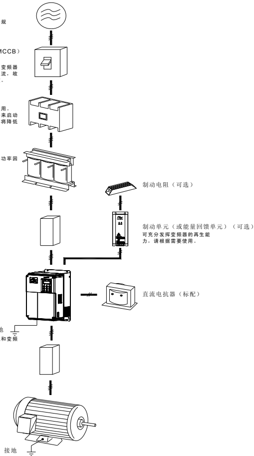
与外围机器的连接示例
