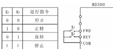
图6-3 两线式运转模式
