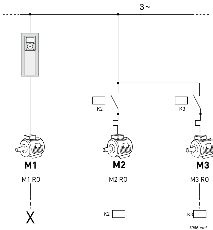
图 104 M1-3 RO = 来自继电器的电机控制，X = 未使用
