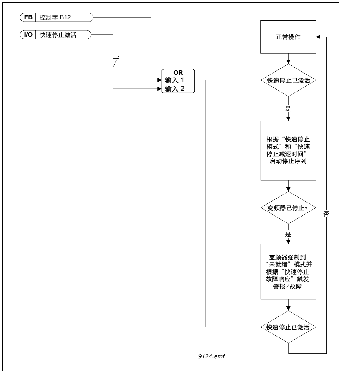
图80 快速停止逻辑
