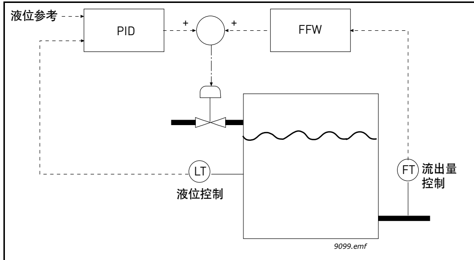
图 86 前馈控制
