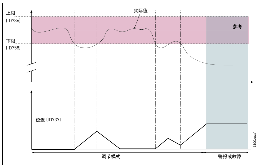
图 88 反馈监控
