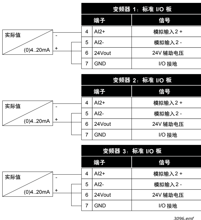
图 100 各个反馈传感器的接线示意
