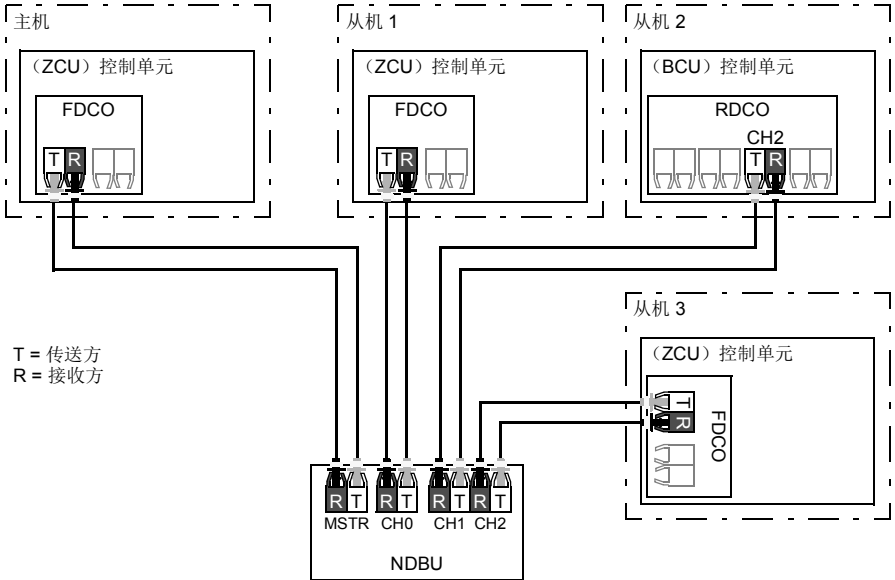
主 / 从光纤电缆的星形配置 (1)
