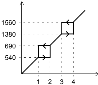
22.01 速度给定值 (rpm) (功能的输出)
